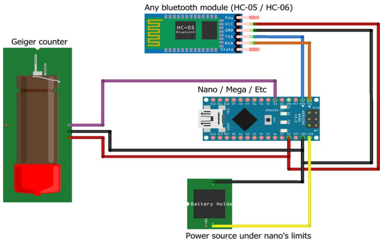
PLANO ESQUEMATICO
